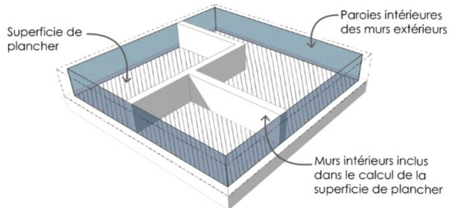
Figure 3. Mesure de la superficie de plancher d'un bâtiment
