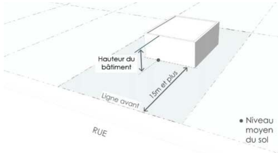
Figure 5. Mesure de la hauteur d'un bâtiment implanté à 15 m et plus de la ligne avant
