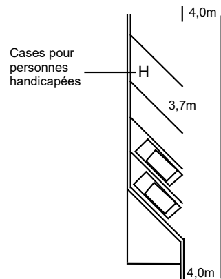
STATIONNEMENT À 60°
