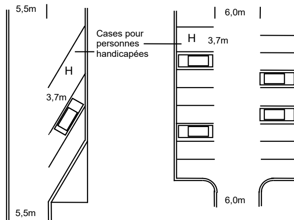
STATIONNEMENT À 60°
