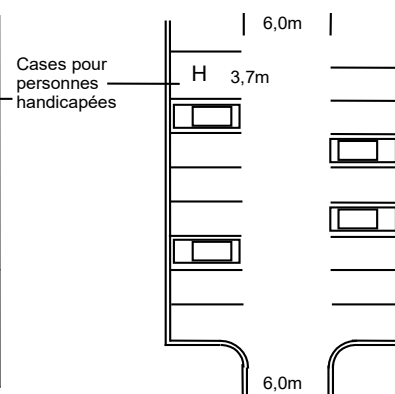
STATIONNEMENT À 90°
