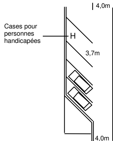
STATIONNEMENT A 60°
